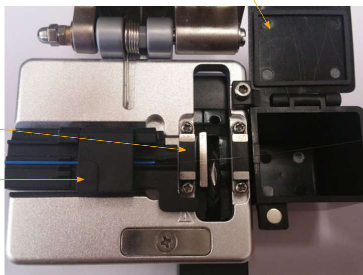
Detalle cortadora con fibra óptica lista para el corte
